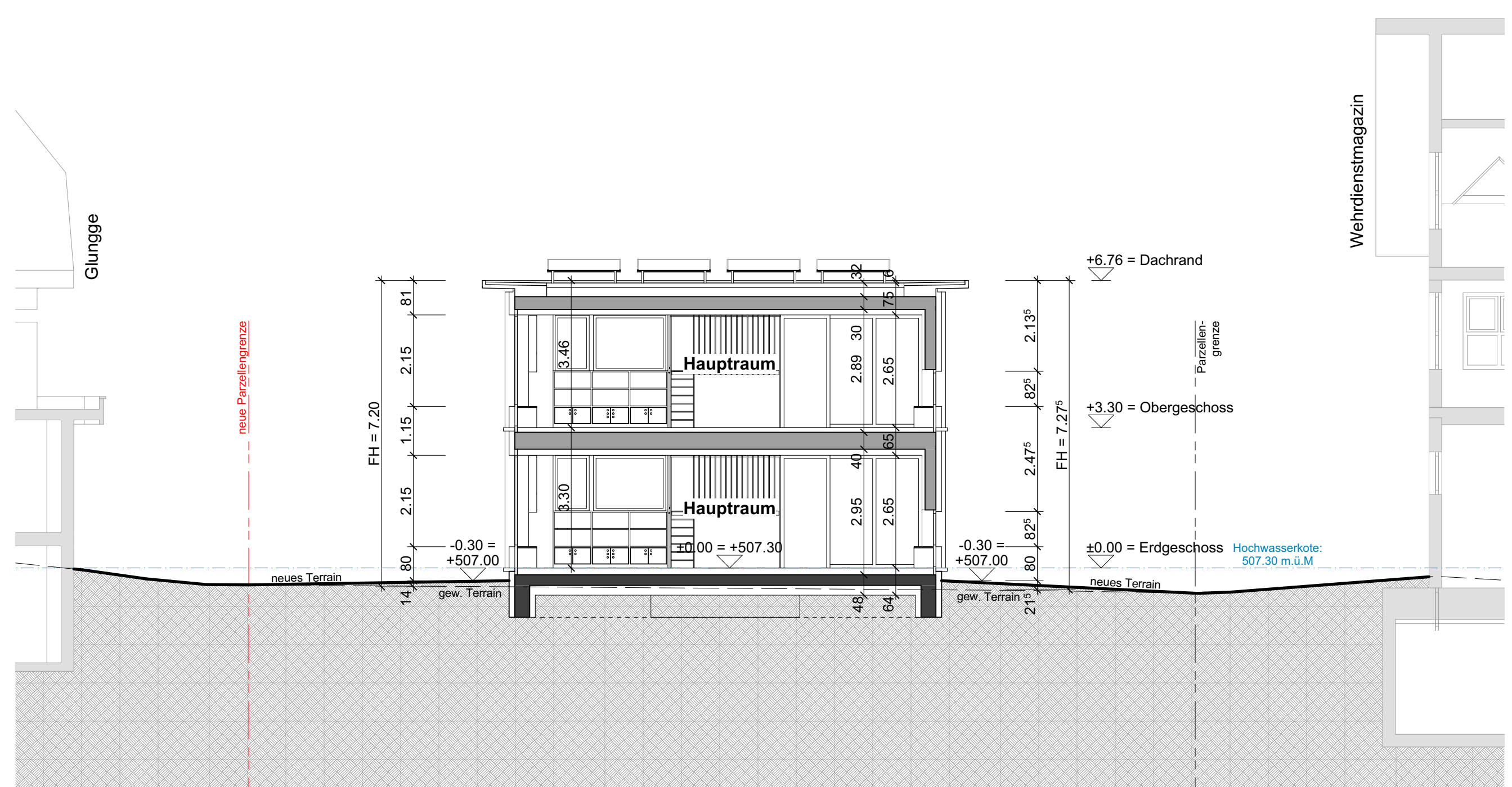
Schnitt 1-1
